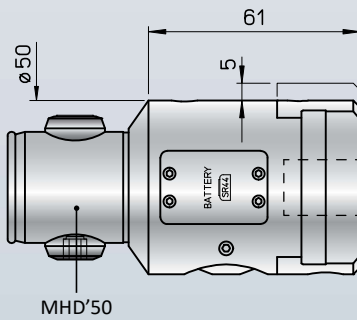
TRE 50 IP69K \varnothing .10~5.59
